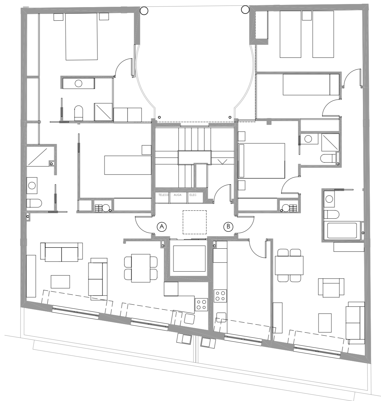
PLANTA ÁTICO
